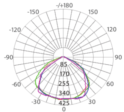
Рисунок 3. Крива сили світла світлодіодних джерел світла
